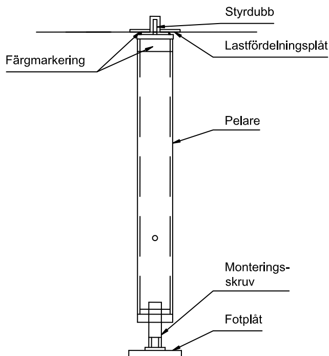
Figur T11-107a. Vy av monterbar pelare med färgmarkering.
